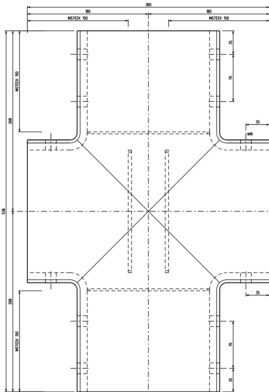
VOORAANZICHT
