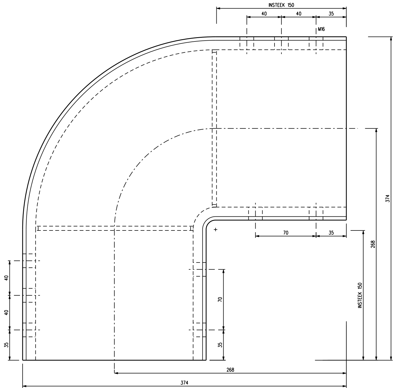
VOORAANZICHT
