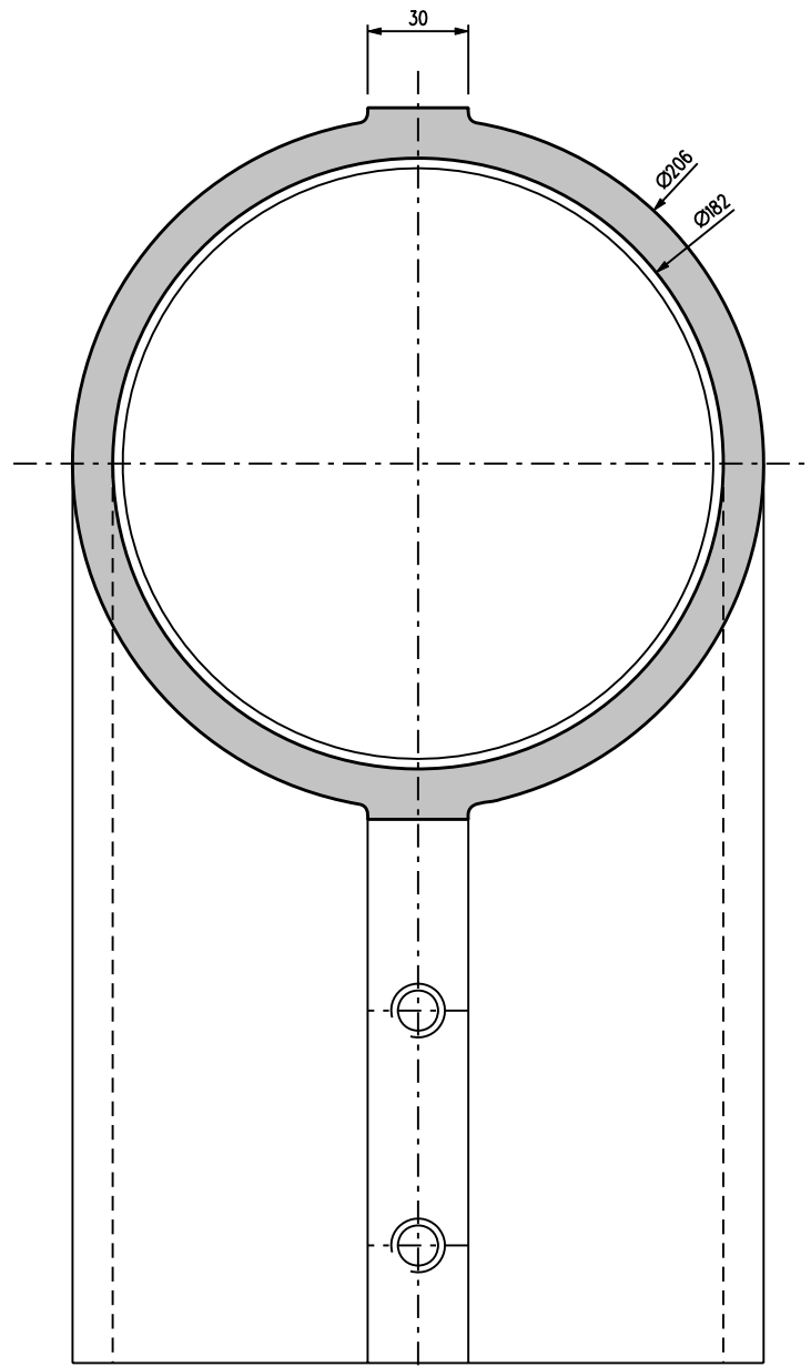
ZIJAANZICHT LINKS
