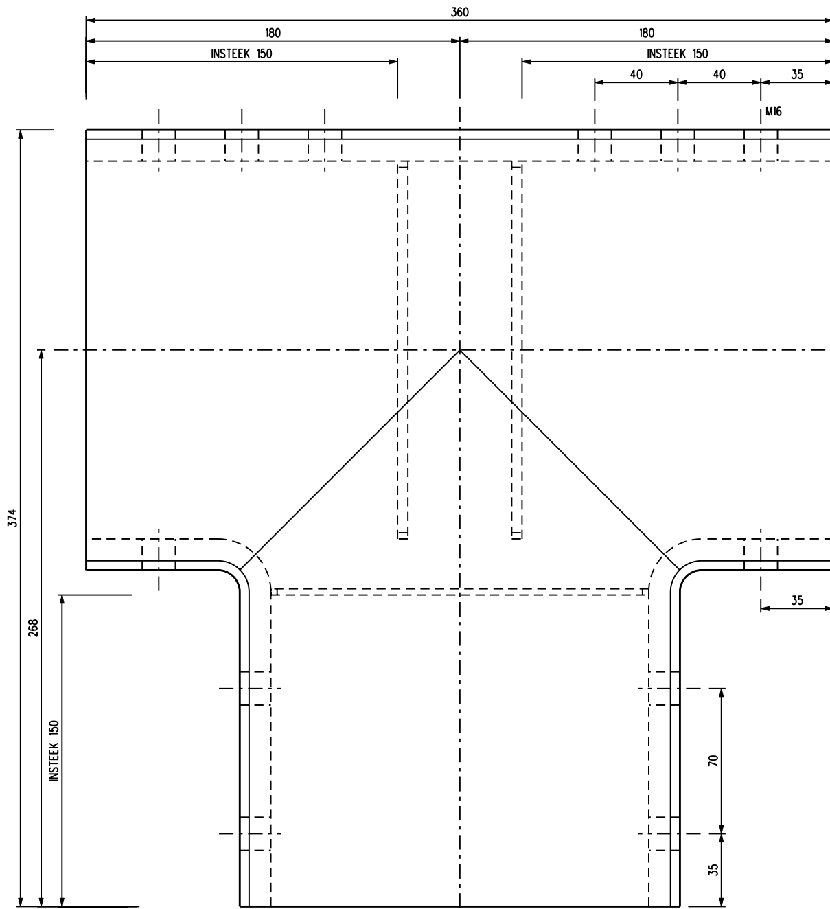
VOORAANZICHT
