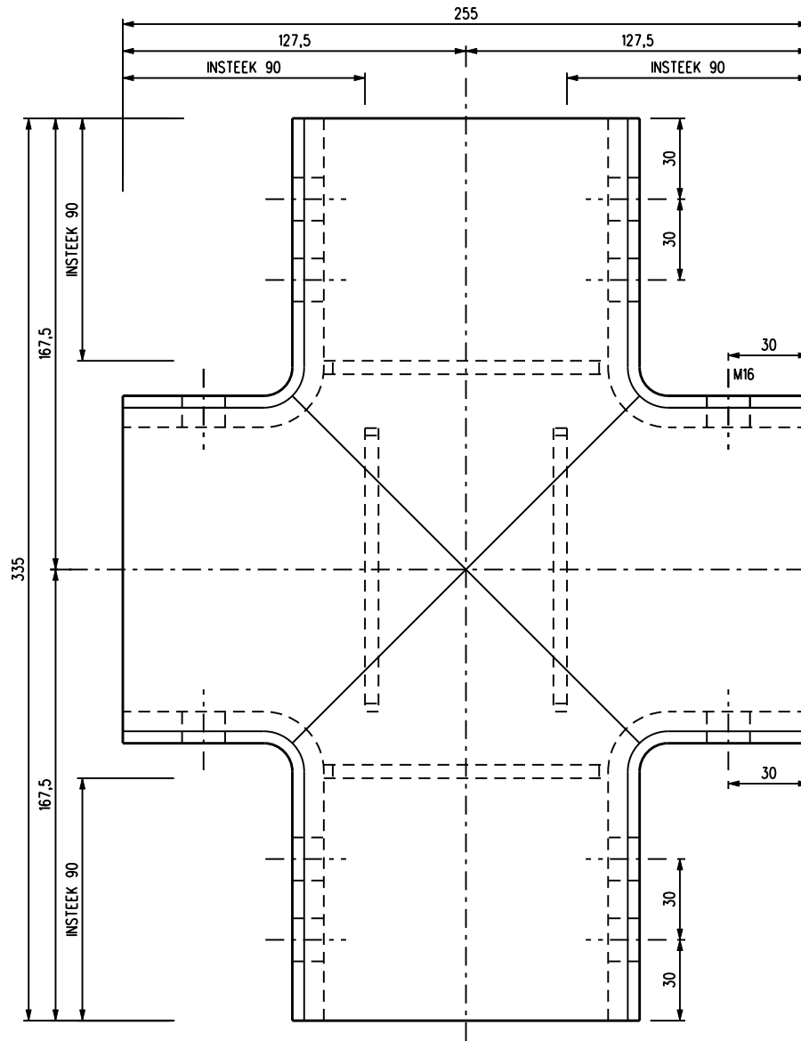
VOORAANZICHT KRUISSTUK TYPE 2
