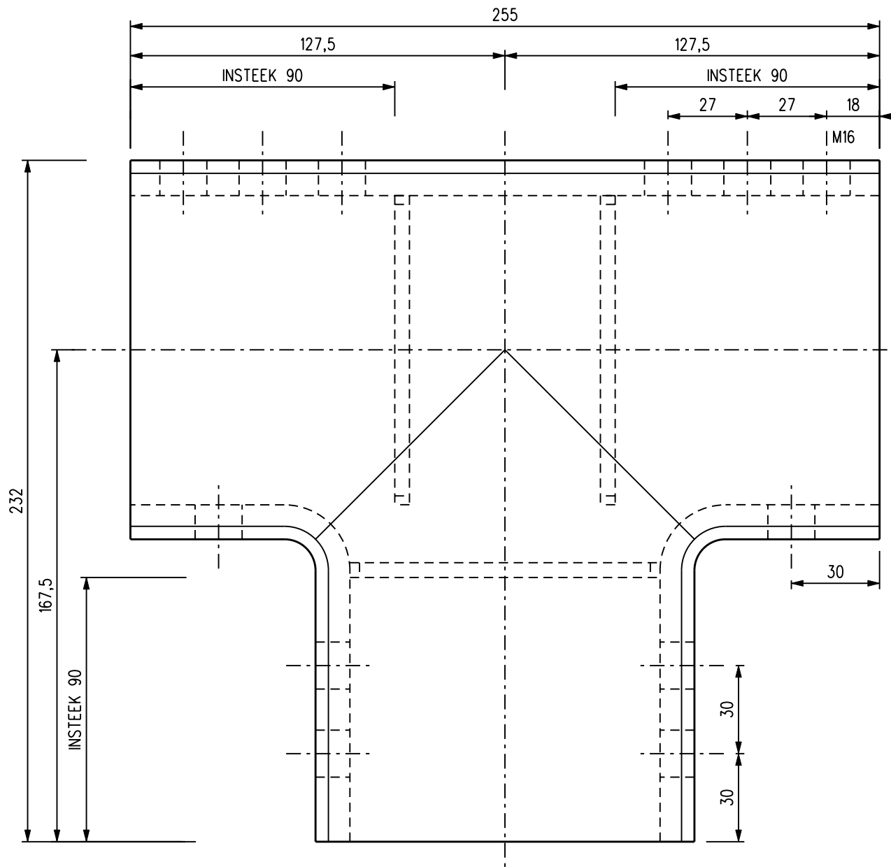
VOORAANZICHT
