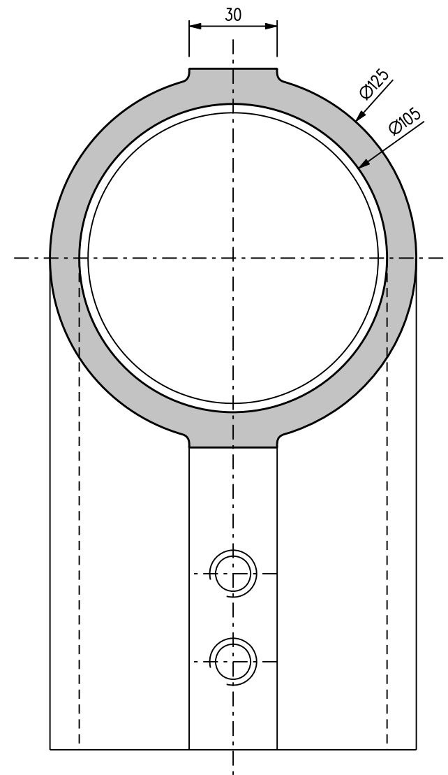
ZIJAANZICHT LINKS
