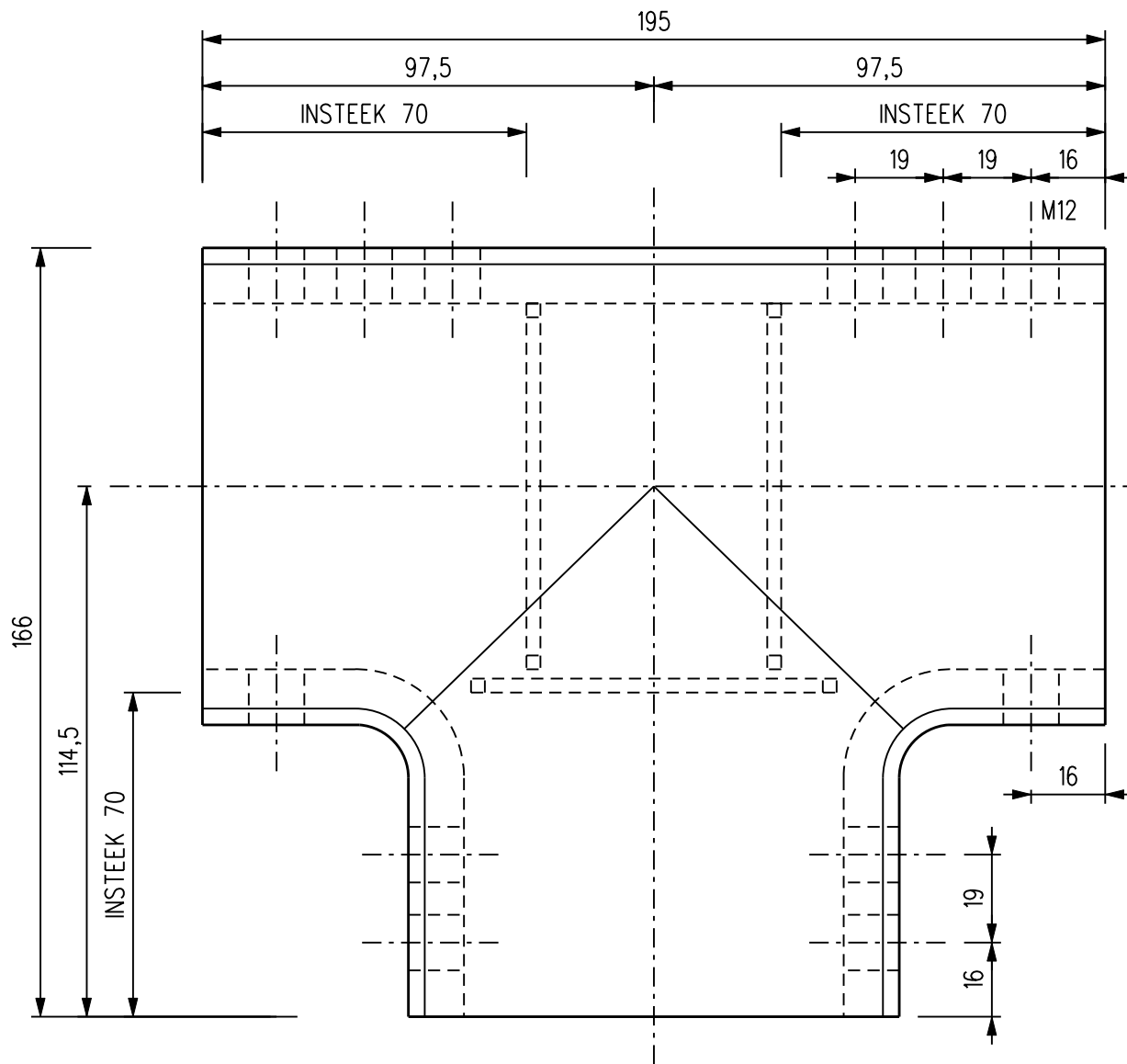
VOORAANZICHT
