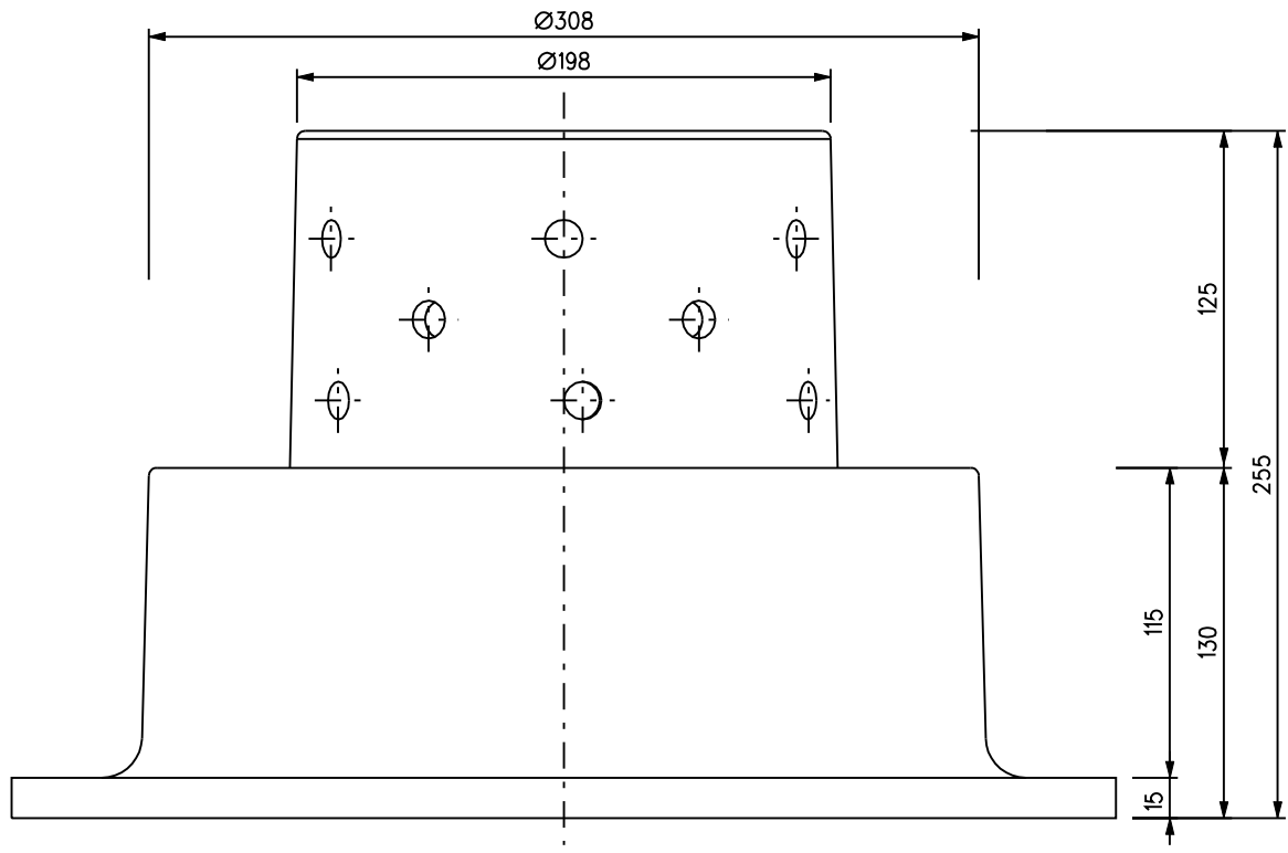
VOORAANZICHT
