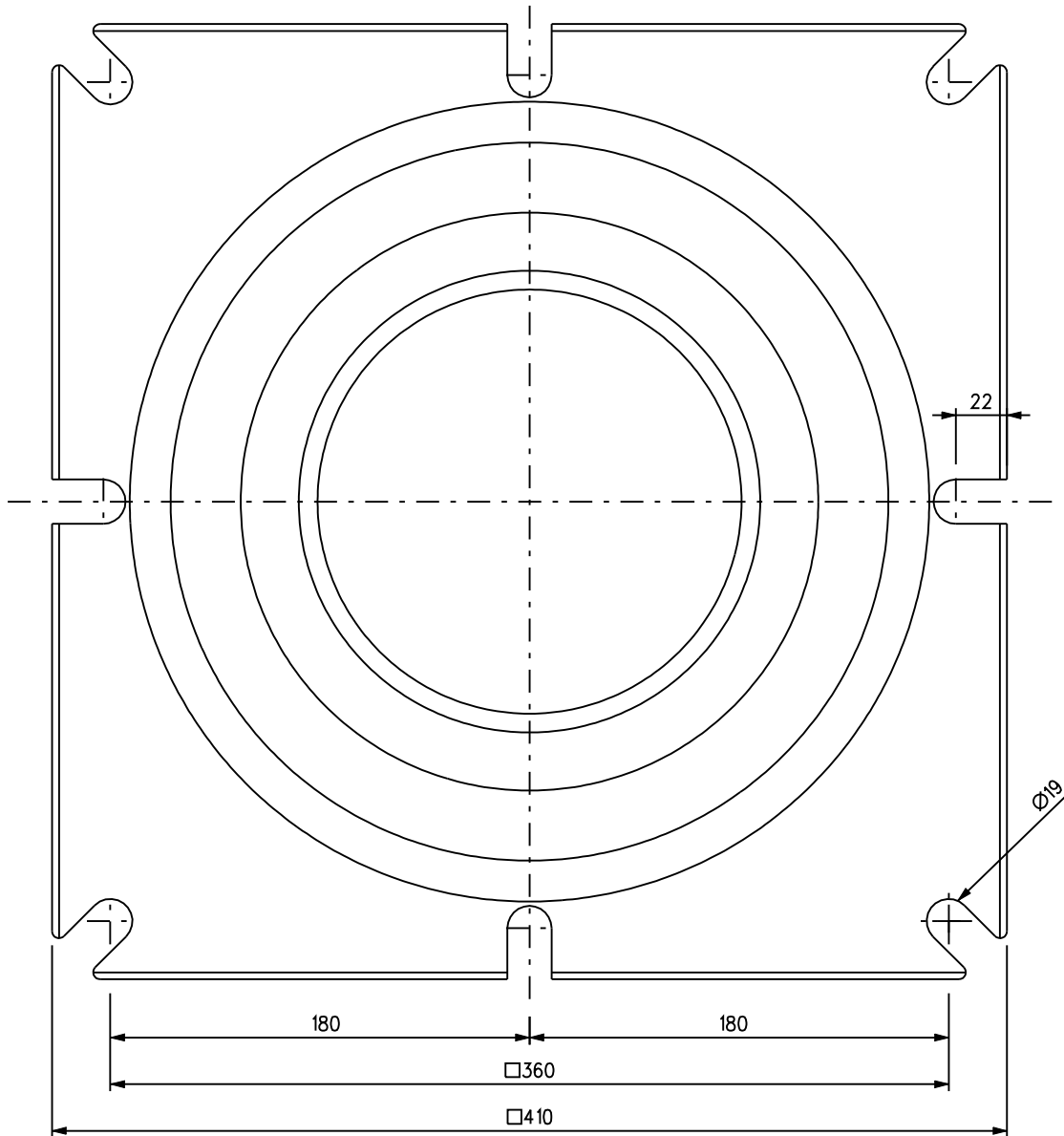
BOVENAANZICHT SOFTSTOP TYPE 3
